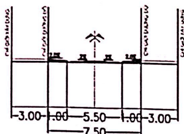
MẶT CÁT 2-2
