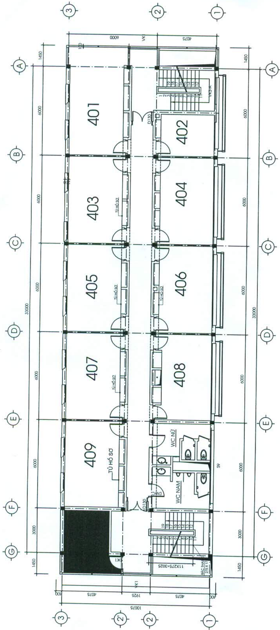
MẶT BẰNG TẦNG 4
